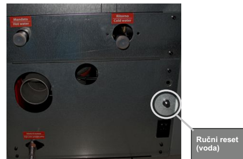
Slika 7. Sigurnosni termostat
