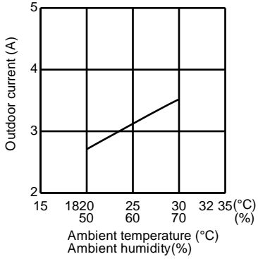
MUZ-HJ60VA
