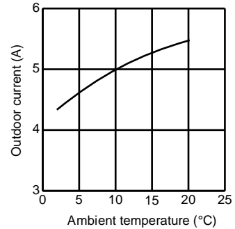
MUZ-HJ50VA
