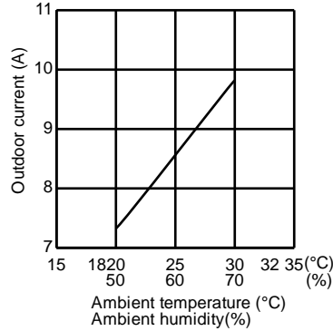
MUZ-HJ71VA
