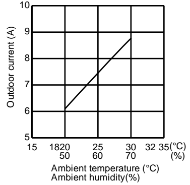
MUZ-HJ50VA
