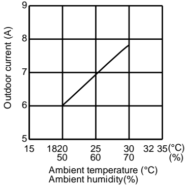
MUZ-HJ60VA
